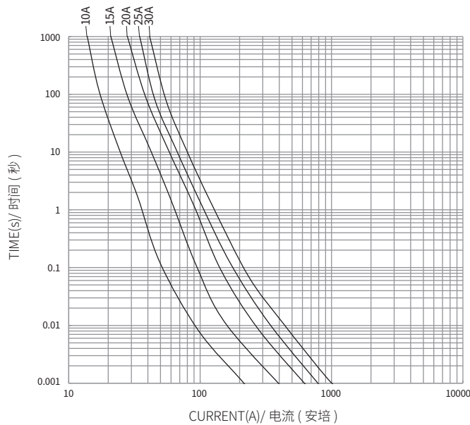
HC100EV-T 系列 平均 I-T 曲线图 (仅供参考) AVERAGE I-T CHARACTERISTICS CURVE (FOR REFERENCE)
